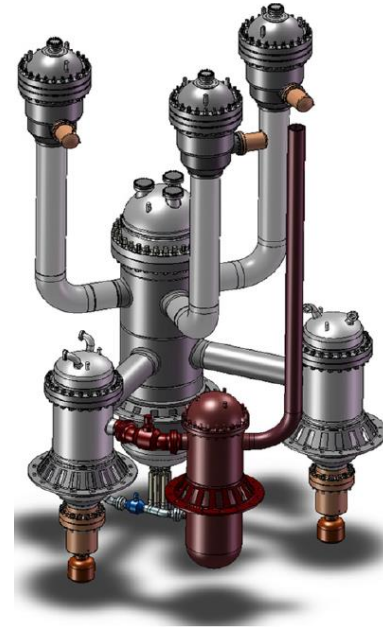
ALLEGRO 75 MW
