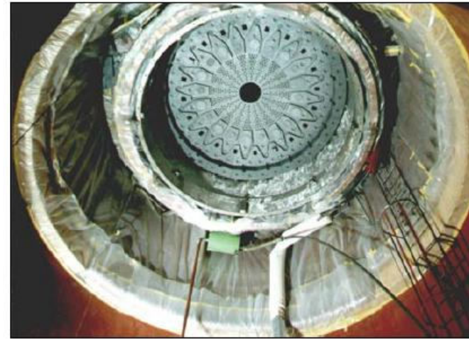
Top Reflector
