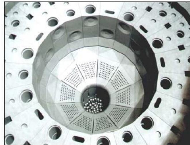
Bottom Reflector
