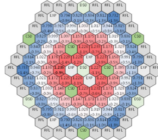
EOC (500 EFPD)
