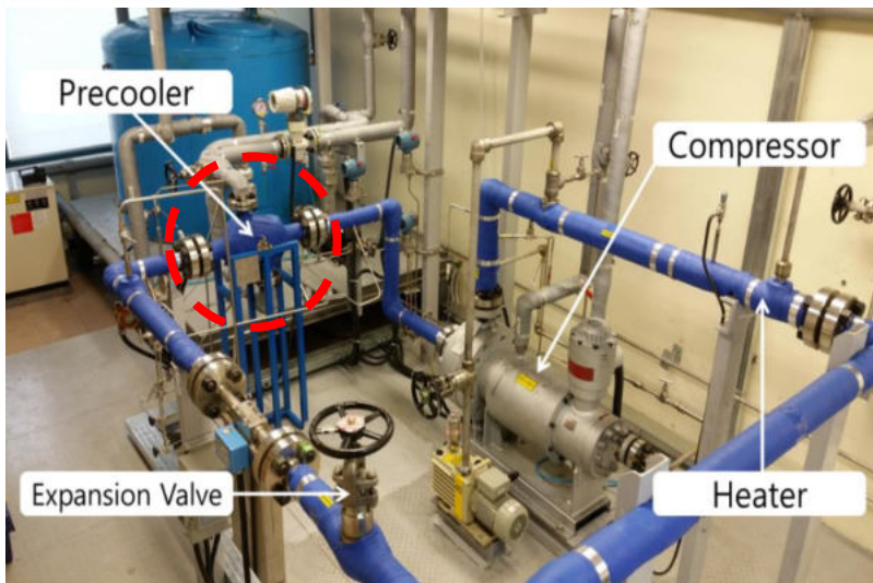
<KAIST-SCO2PE>
