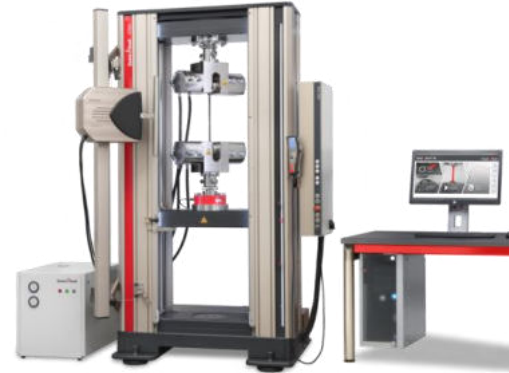
Zwick/Roell Z200 AllroundLine
