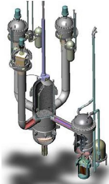
ETDR 50 MW
